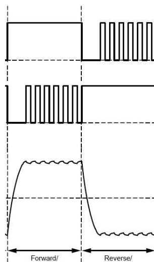
FIGURE 8 – Hacheur A4950 : Chronogrammes de fonctionnement
